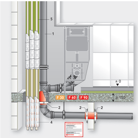
Beispiele für Abschottungen in Massivdecken und -wänden.
