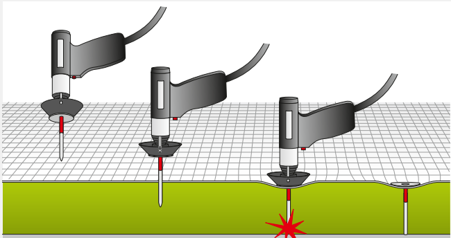
Befestigung mit Clip-Pin-Schweißstiften
